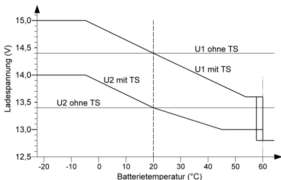
Ladeprogramm „Lead Acid DIN“, Kennlinie IU1oU2
