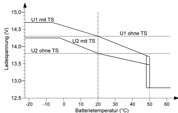
Ladeprogramm „GEL“, Kennlinie IU1oU2
