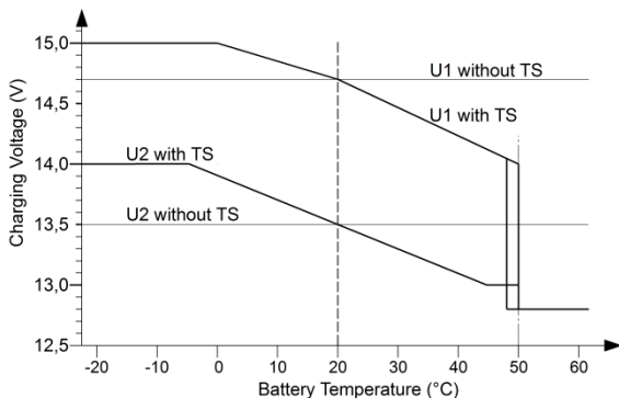
Ladeprogramm „AGM2“, Kennlinie IU1oU2
