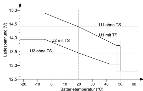
Ladeprogramm „AGM1“, Kennlinie IU1oU2
